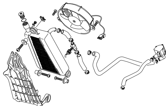
REFRIGERACIÓN - COOLING SYSTEM
