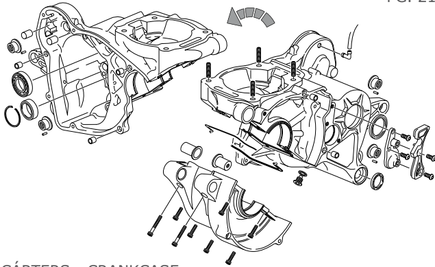
CÁRTERS - CRANKCASE
