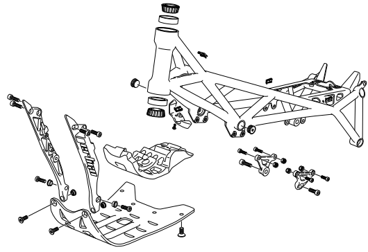
BASTIDOR - FRAME
