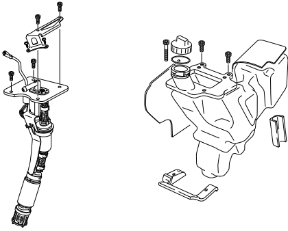
DEPÓSITO DE GASOLINA - FUEL TANK
