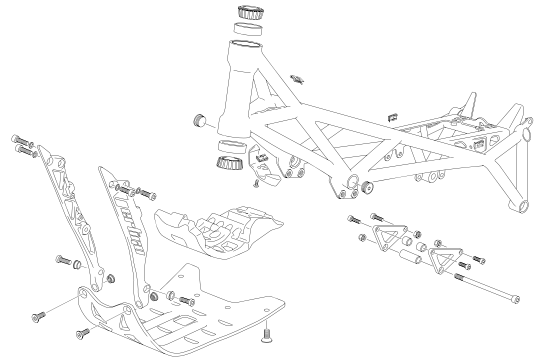
BASTIDOR - FRAME
