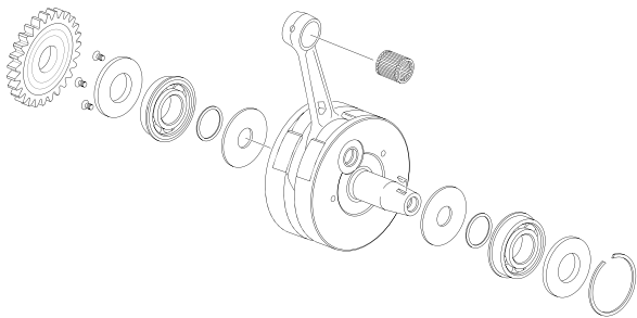
CIGÜEÑAL - CRANKSHAFT
