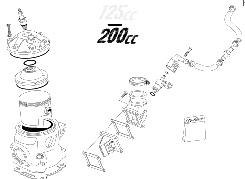
CUERPO INYECCIÓN - INJECTION BODY
