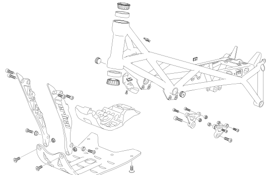
BASTIDOR - FRAME
