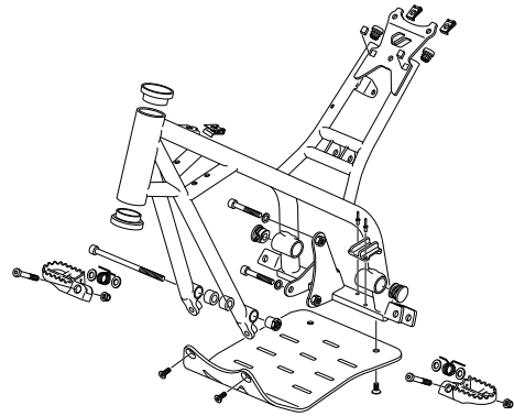
BASTIDOR - FRAME
