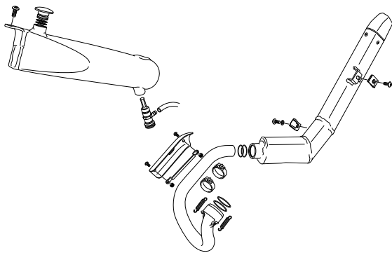
ESCAPE-DEPÓSITO - EXHAUST-TANK
