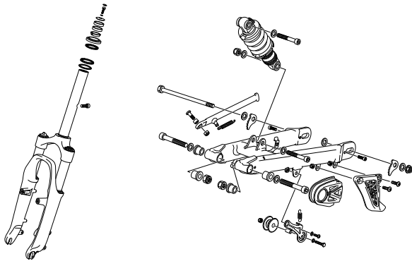
AMORTIGUACIÓN - SUSPENSION
