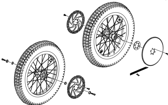
RUEDAS - WHEELS
