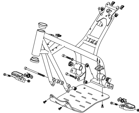
BASTIDOR - FRAME
