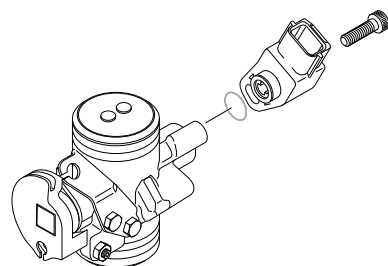
CUERPO INYECCIÓN - INJECTION BODY
