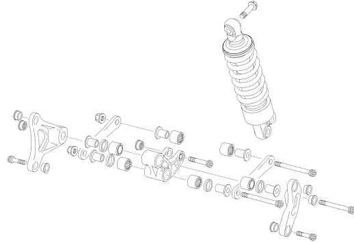
AMORTIGUACIÓN - ROCKER
