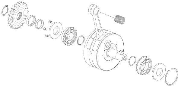
CIGÜEÑAL - CRANKSHAFT
