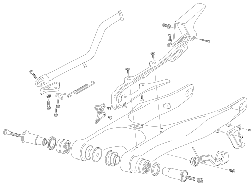
BASCULANTE - SWINGARM
