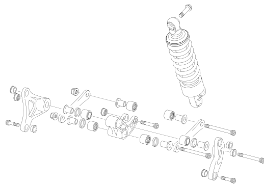
AMORTIGUACIÓN - ROCKER
