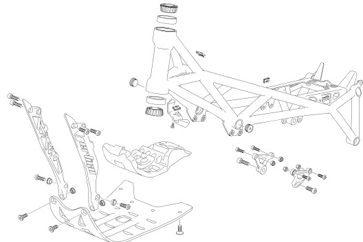
BASTIDOR - FRAME
