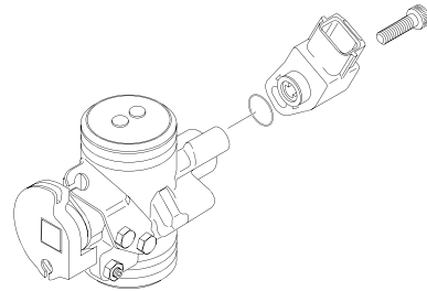
CUERPO INYECCIÓN - INJECTION BODY
