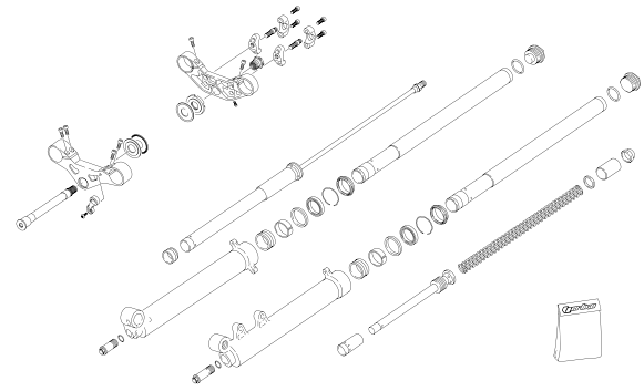
HORQUILLA SUSPENSIÓN - FORK
