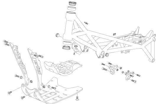
BASTIDOR - FRAME
