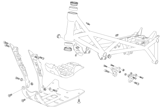
BASTIDOR - FRAME
