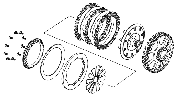
EMBRAGUE - CLUTCH
