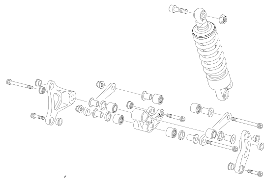
AMORTIGUACIÓN - ROCKER
