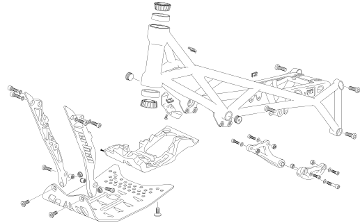
BASTIDOR - FRAME
