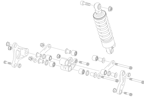
AMORTIGUACIÓN - ROCKER
