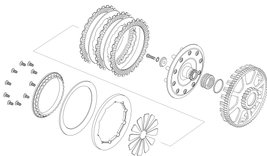
EMBRAGUE - CLUTCH
