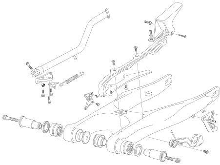
BASCULANTE - SWINGARM
