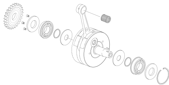
CIGUEÑAL - CRANKSHAFT
