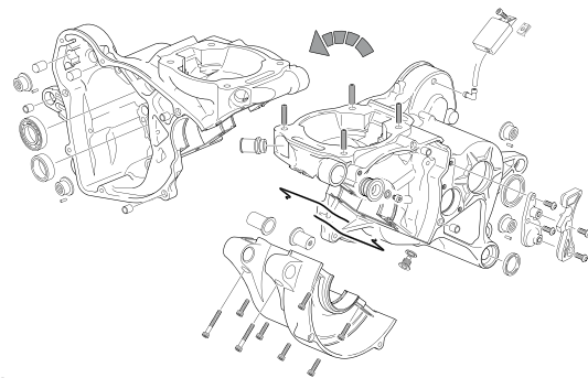
CÁRTERS - CRANKCASE
