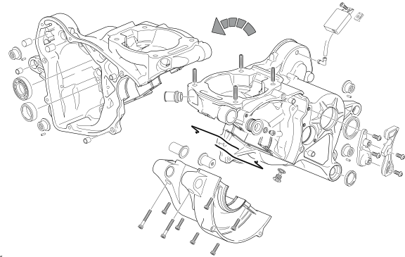
CÁRTERS - CRANKCASE
