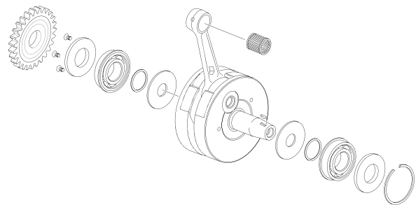
CIGUEÑAL - CRANKSHAFT
