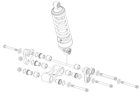
AMORTIGUACIÓN - ROCKER
