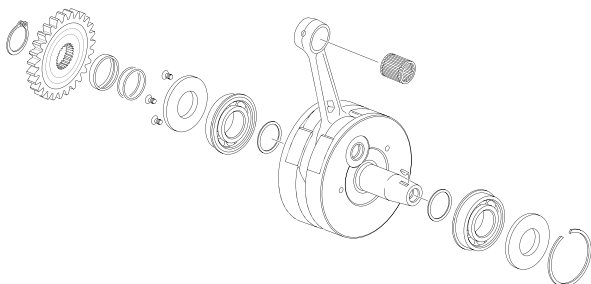
CIGUEÑAL - CRANKSHAFT
