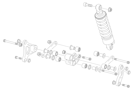
AMORTIGUACIÓN - ROCKER
