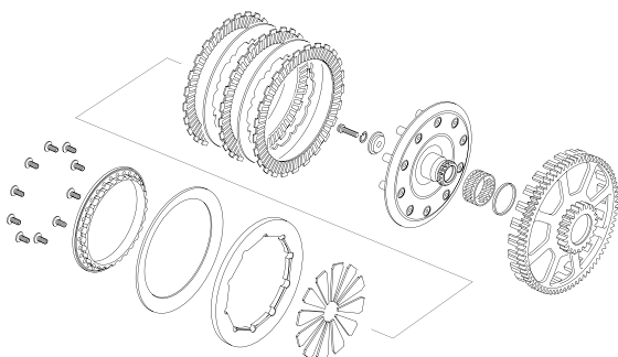
EMBRAGUE - CLUTCH
