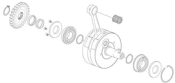
CIGUEÑAL - CRANKSHAFT
