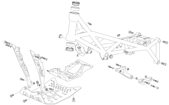
BASTIDOR - FRAME
