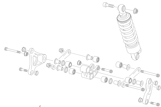
AMORTIGUACIÓN - ROCKER
